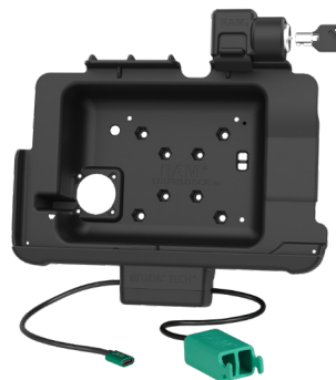
Tough Latching 仕様 電源・周辺機器コネクタ・キー付きロックを接続した状態でも使用可能 頻繁にドッキングや取り外しを行う場合に最適です。
