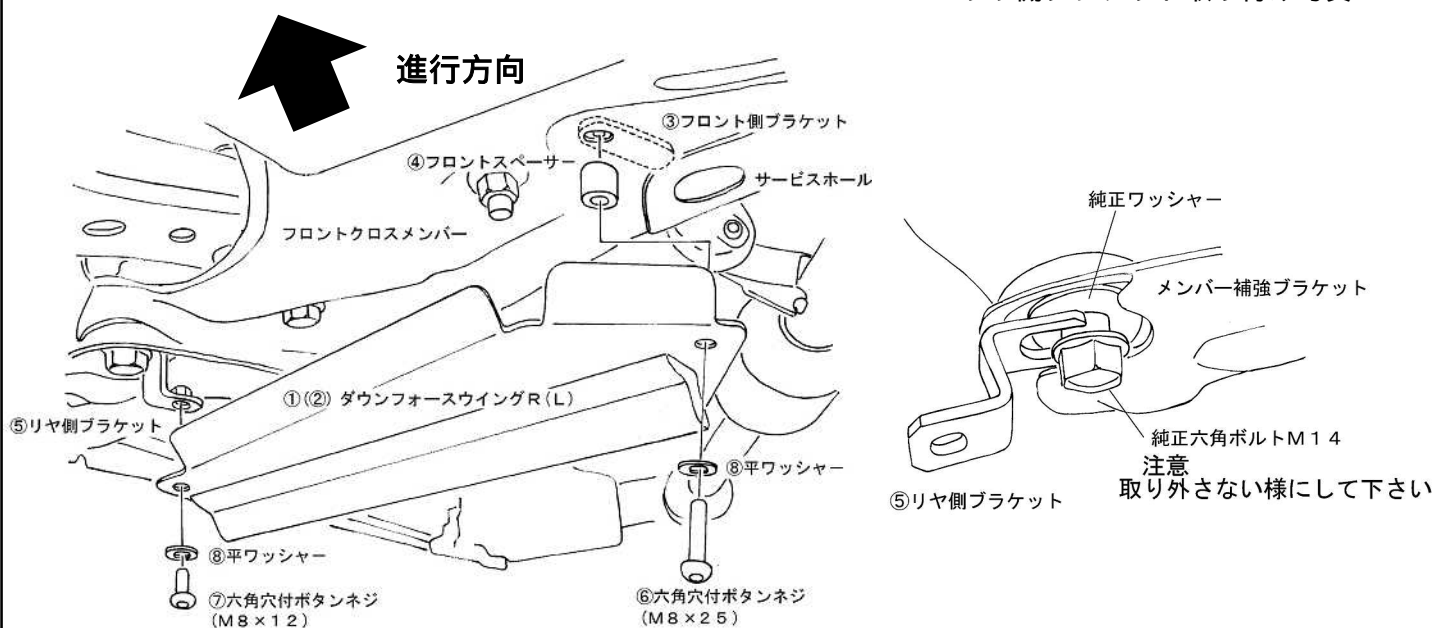
リヤ側ブラケット取り付け写真
