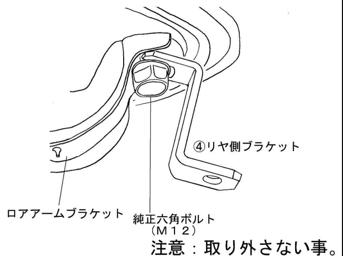
リヤ側ブラケット取り付け図
