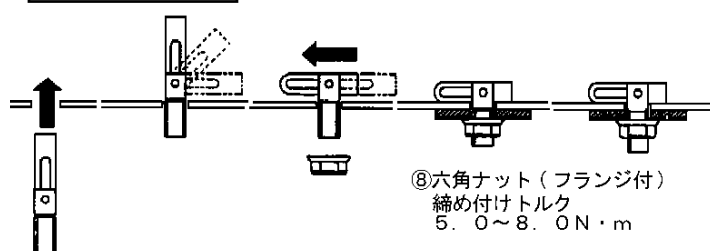
ITボルト組付け手順
