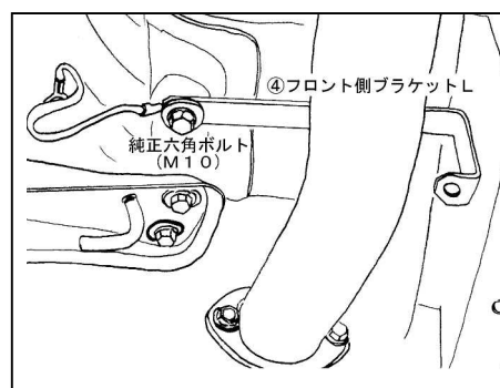
左側ブラケット取り付け図
