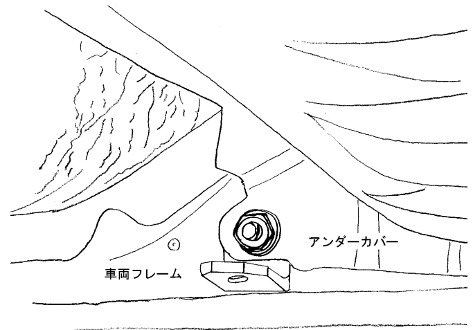
リヤ側ブラケット取り付け位置
