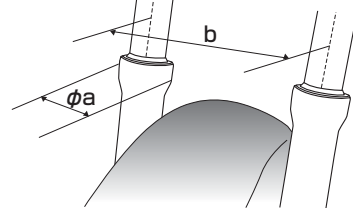
a:リペアフォークブラケットセット(キャップボルト付属)
